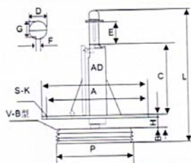
冷却塔专用减震器(方塔)
