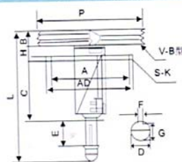
冷却塔专用减震器(圆塔)
